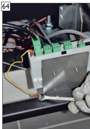
Ringöse des Erdungskabels der Steuerung mit der Befestigungsschraube am Blendrahmen befestigen. ACHTUNG! Befestigungsschraube muss von unten in den Blendrahmen geschraubt werden!
