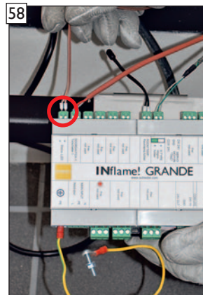
Anschlussstecker der Status-LED in die Steuereinheit einstecken.
