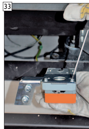
Stellmotorhalterung für Gleitlager mit den Befestigungsschrauben am Stellmotor montieren.
