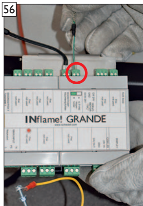
Anschlussstecker des Abgas-temperatursensors in die Steuereinheit einstecken.
