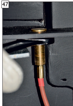
Türkorkontaktschalter mit Haltemutter fixieren.
