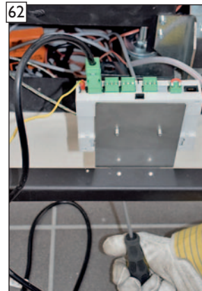
Haltewinkel der Steuereinheit in die Befestigungsschrauben im Blendrahmen einstecken und festziehen.
