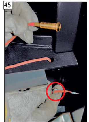
Verbindungskabel durch die Öffnung des Türkontaktschalters fädeln und Haltemutter des Türkontaktschalters anschließend auffädeln.
