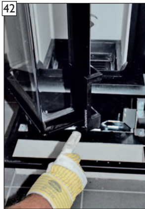
Montageposition für den Türkontaktmagnet an der Gerätetür.
