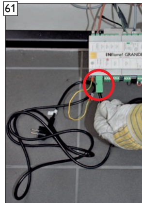
Anschlussstecker des 230 V-Netzkabels in die Steuereinheit einstecken.
