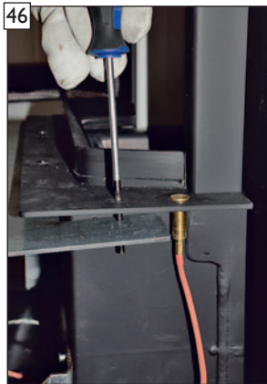
ACHTUNG! Halteblech muss max. gelöst werden um die Haltemutter mit Werkzeug zu erreichen!
