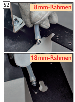
Status-LED mit Leuchtmittel nach unten zeigend in Blendrahmenaufnahme einstecken und ...
