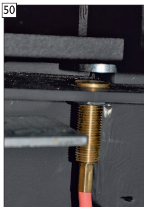
Fertigansicht Montierter Türkorkontaktschalter bei geschlossener Tür mit Türkorkontaktmagnet.
