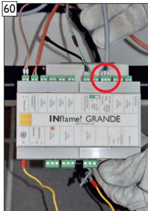
Anschlussstecker des Stellmotor-Verbindungskabels in die Steuereinheit einstecken.
