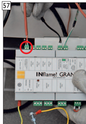
Anschlussstecker des Türkontaktschalters in die Steuereinheit einstecken.
