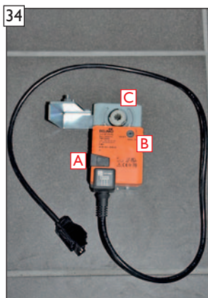
A - Freilaufaste B - Drehrichtungsschalter C - Stellmotorwelle
